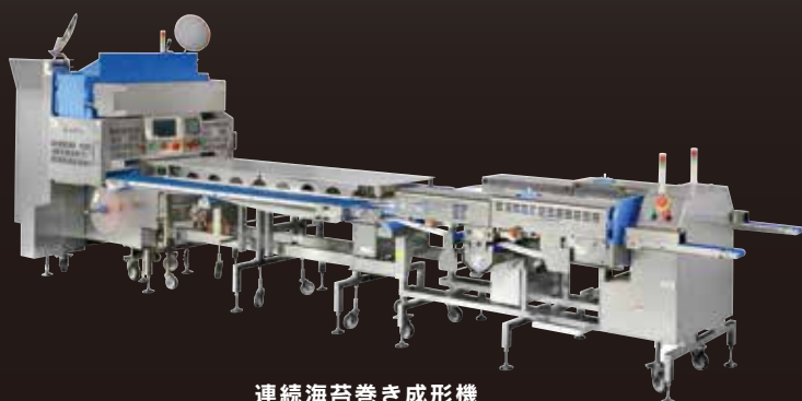
連続海苔巻き成形機 SVR-SAE-W50
